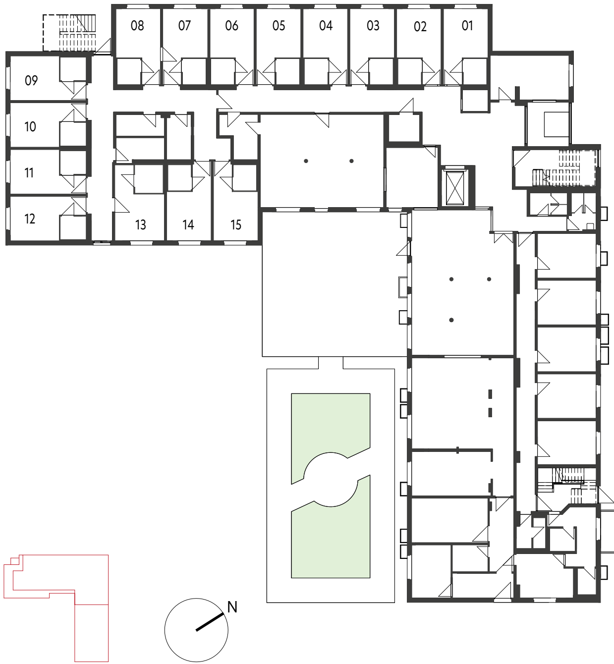
ERDGESCHOSS
